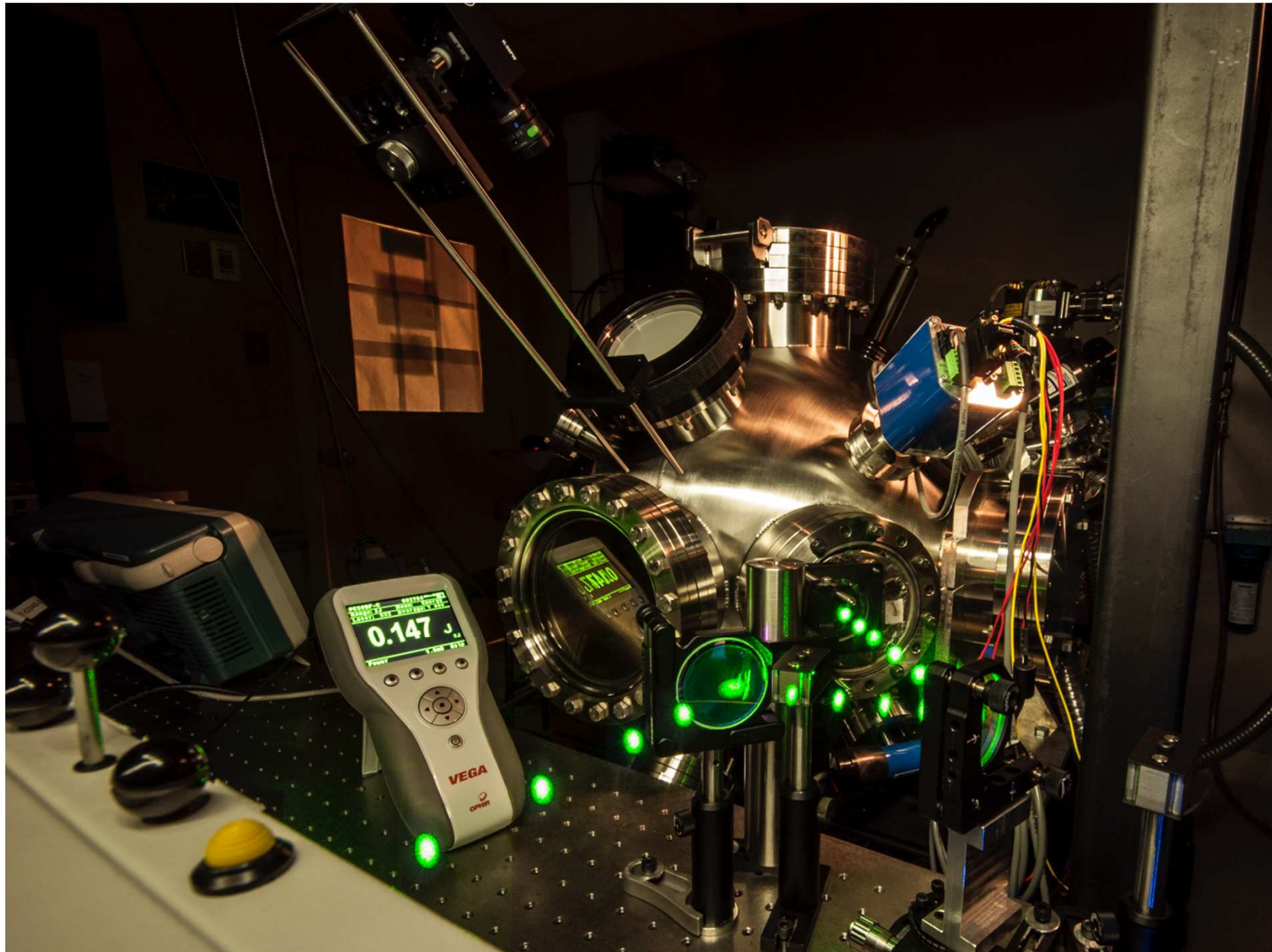
Aperçu du laser en fonctionnement à la longueur d'onde 532 nm à une cadence de 5Hz. Les impulsions qui sortent du laser sont redirigées vers la chambre à vide à l'aide de deux miroirs puis concentrées avec une lentille vers une cible placée au centre de la chambre. Photo prise par Maxime Boudreau.
